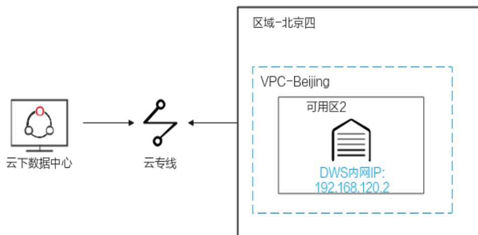
图 6-5 云专线访问
