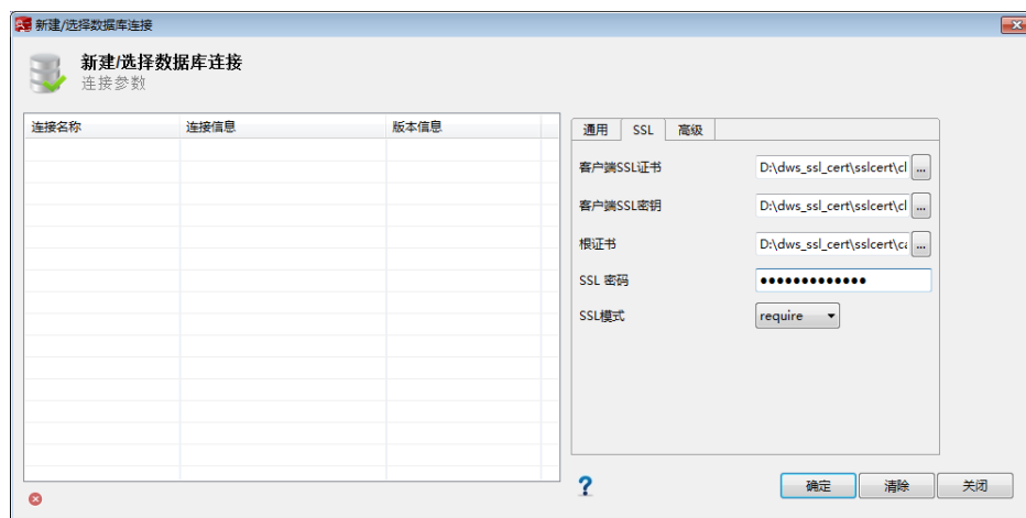
图 4-3 配置 SSL 参数
