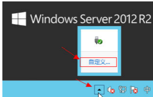
图 2-29 单击“自定义”
