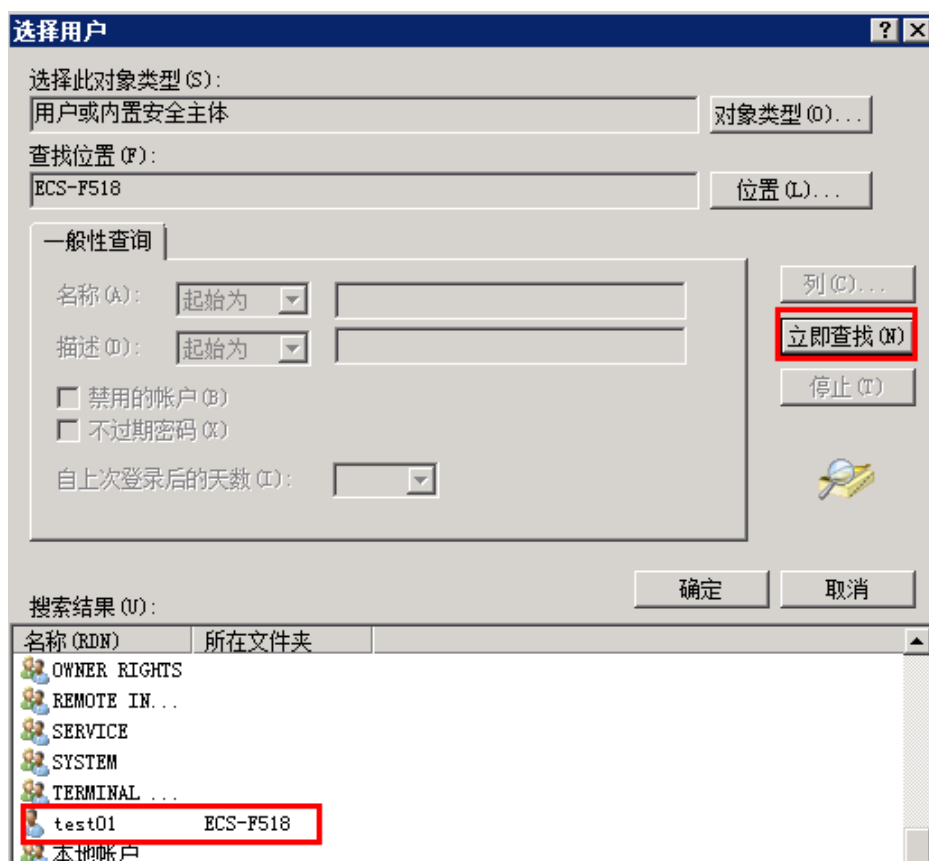
图 9-20 选择用户
