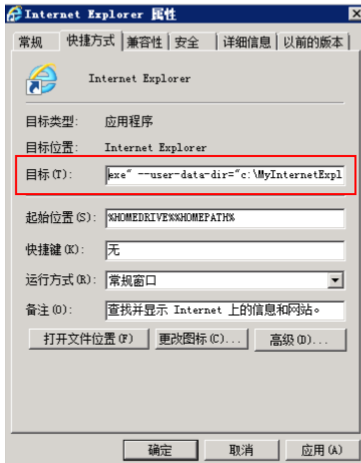
图 9-44 浏览器属性
