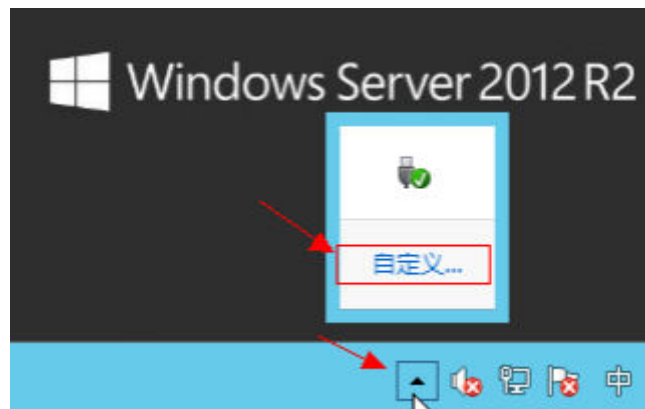
图 2-40 单击“自定义”
