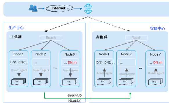
图 3-21 双集群容灾
