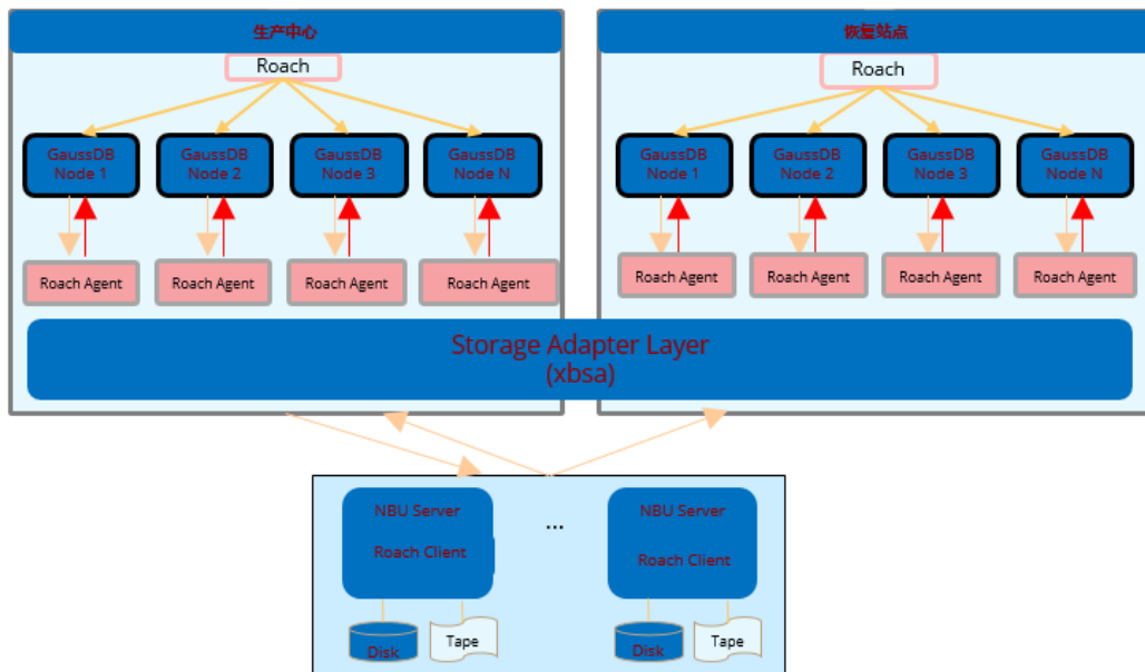
图 3-20 备份恢复生态对接架构
