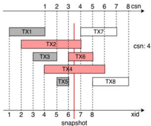
图 3-6 CSN 的更新以及与 XID 的映射关系
