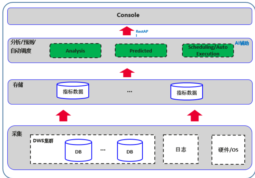
图 4-9 DMS 架构
