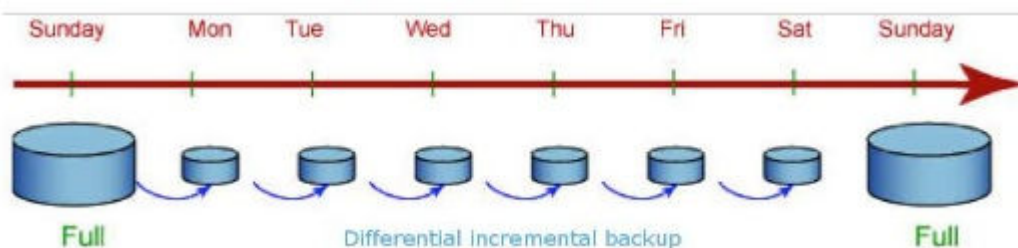
图 3-19 自动快照的备份与恢复策略
