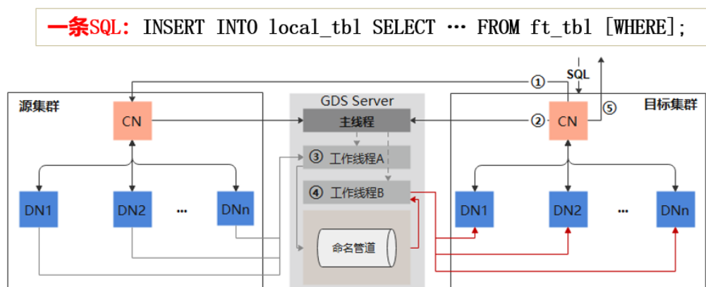
图 3-11 拉取方式
